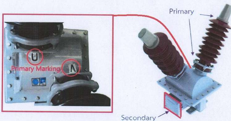
รูปที่ 13 ตัวอย่างเครื่องหมายและฉลากบนจุดต่อสายด้าน Primary
