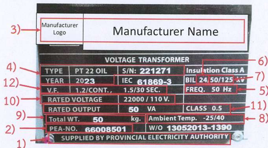
รูปที่ 13 ตัวอย่างเครื่องหมายและฉลากบน Nameplate ของ H.V. VT
