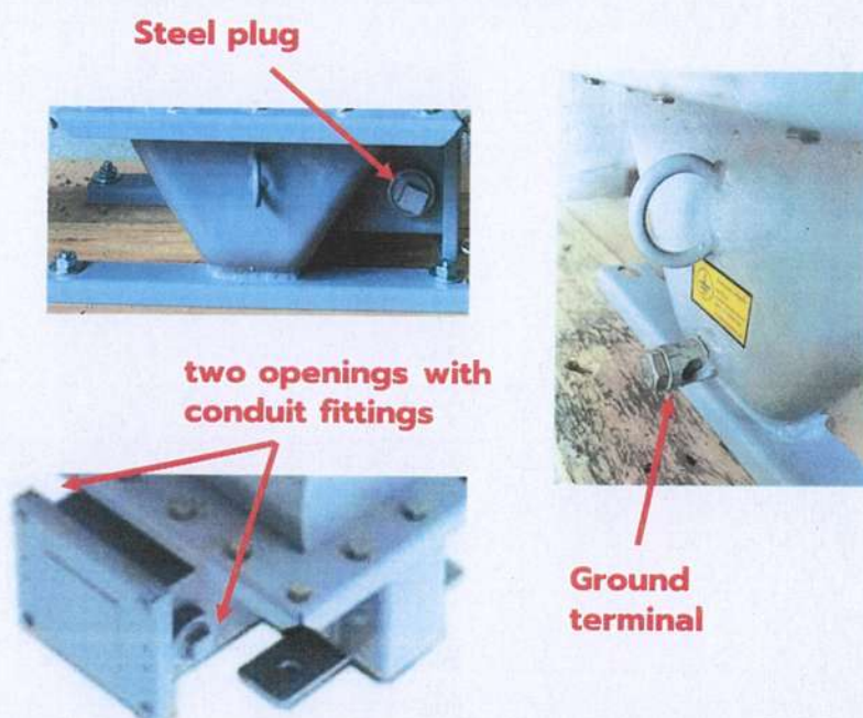
รูปที่ 11 ตัวอย่างกล่องจุดต่อสายด้าน Secondary และจุดต่อสายกราวด์
