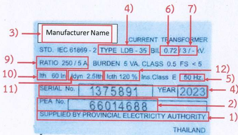
รูปที่ 9 ตัวอย่างเครื่องหมายและฉลากบน Nameplate
