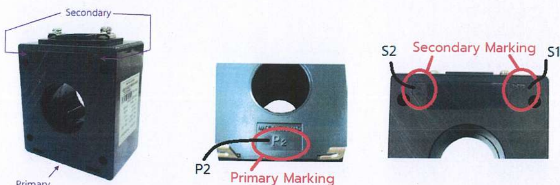
รูปที่ 8 ตัวอย่างเครื่องหมายบนจุดต่อสาย (Terminal marking)
