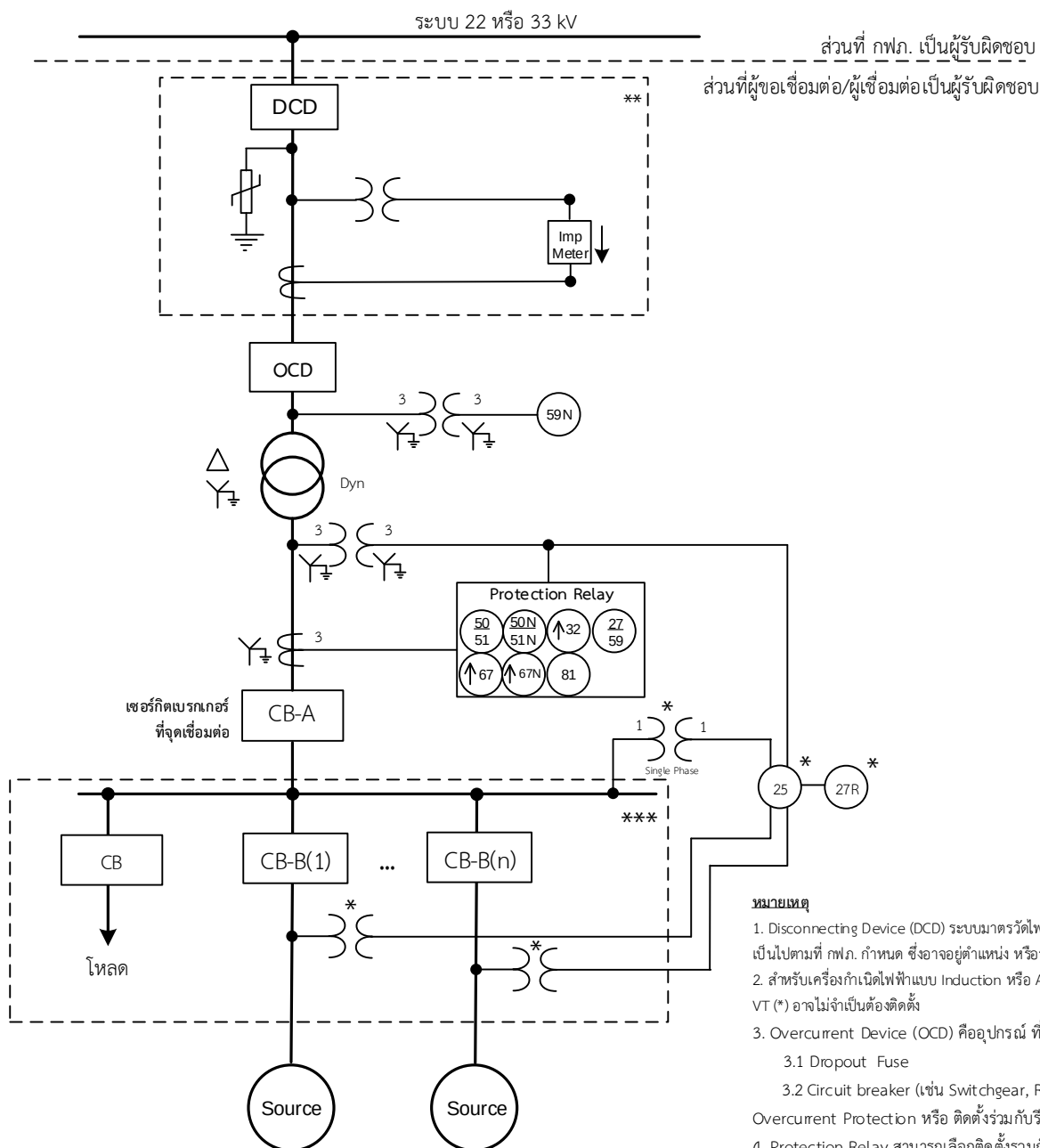
รูปแบบที่ 2.6 การเชื่อมต่อของผู้ใช้ไฟฟ้าที่มีเครื่องกำเนิดไฟฟ้าชนิด Non - Inverter ขนาดพิกัดรวมกันไม่เกิน 1 MW กับระบบ 22 หรือ 33 kV
