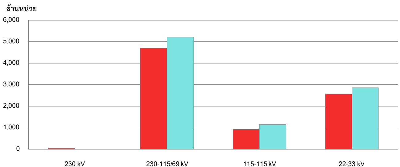
เปรียบเทียบหน่วยซื้อ แยกตามแรงดัน เดือน มิ.ย.52 กับ มิ.ย.53
