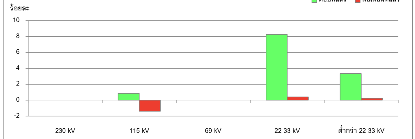
อัตราเพิ่ม(ลด)จำนวนผู้ใช้ไฟฟ้า แยกตามแรงดัน เดือน เม.ย.52 กับ เม.ย.53
