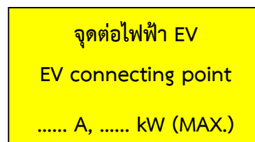
รูปที่ 10 ป้ายแสดงข้อความเตือนสำหรับเต้ารับโหมด 2
