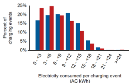
รูปที่ 5-13 รูปแบบพฤติกรรมในการอัดประจุไฟฟ้าของยานยนต์ไฟฟ้าจากการสำรวจของสหรัฐอเมริกา
