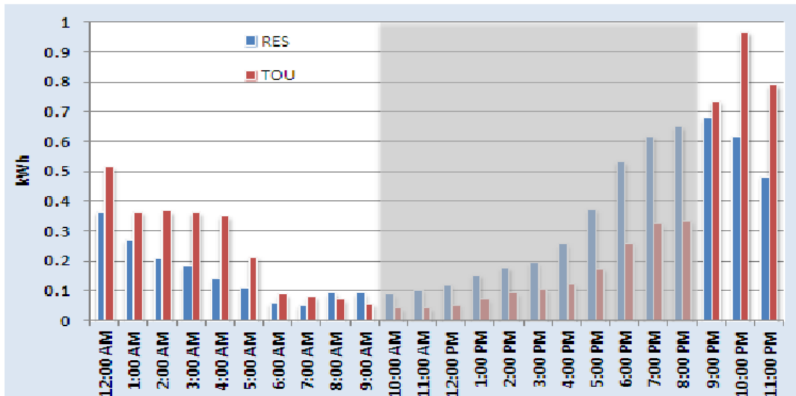
รูปที่ 5-10 รูปแบบการอัดประจุไฟฟ้าของยานยนต์ไฟฟ้า เปรียบเทียบกรณีที่มีการคิดค่าไฟฟ้าแบบ TOU และไม่มีอัตรา TOU ระหว่างวันธรรมดา
