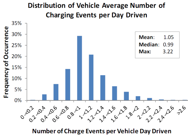
รูปที่ 5-12 จำนวนการอัดประจุต่อการขับขี่ยานยนต์ไฟฟ้าภายใน 1 วัน
