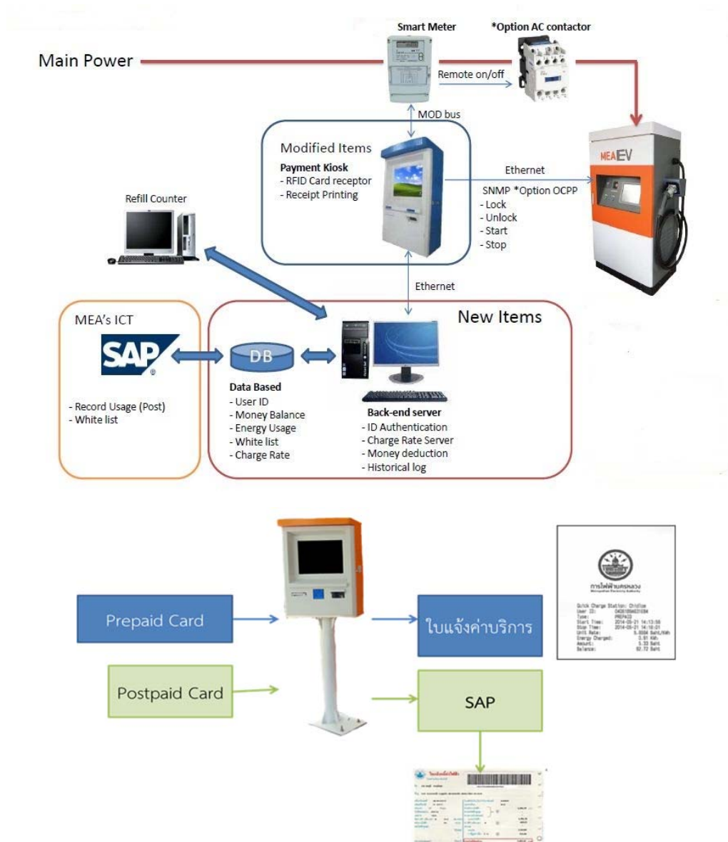
รูปที่ 2-10 ระบบเก็บเงินสำหรับสถานีอัดประจุไฟฟ้าของ กฟน.
