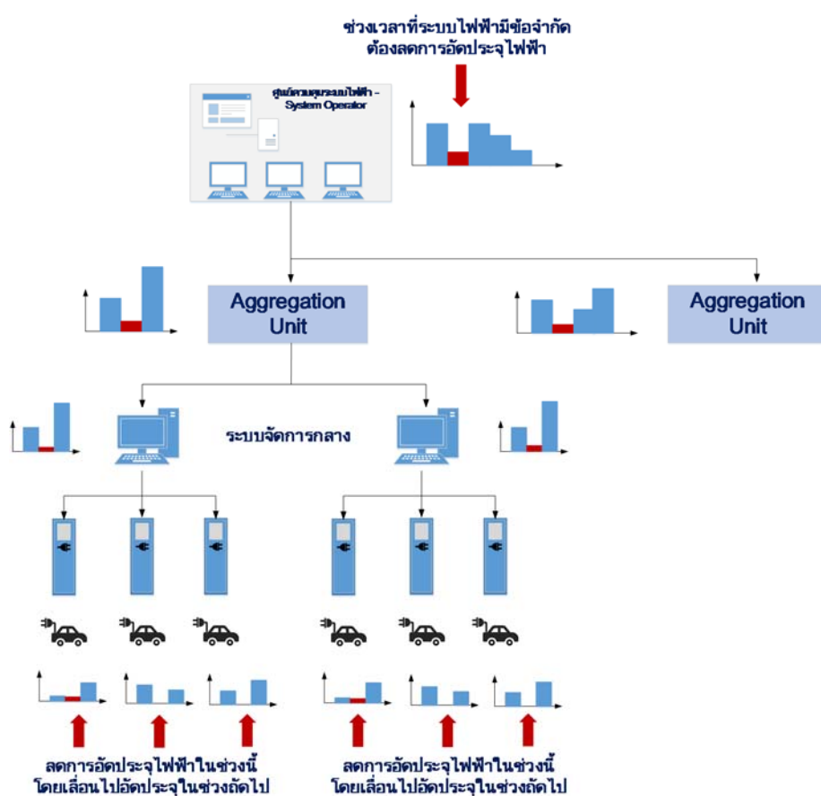
รูปที่ 6-7 การลดการใช้ไฟฟ้าในช่วงเวลาที่มีข้อจำกัด
